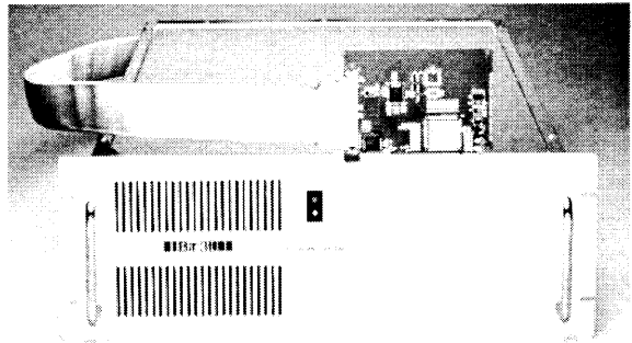
Bit3 DD23 (13スロットPCI拡張シャーシ 19' ラックマウント)
